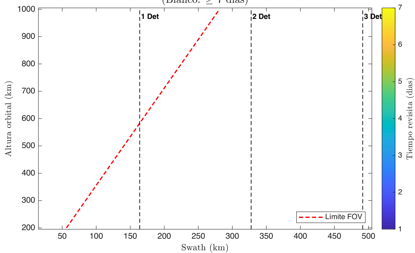
Tiempo Revisita - 1 Satellite(s); 2 Telescopio(s): TMA; Detector 2 (Blanco: \geq 7 dias)
